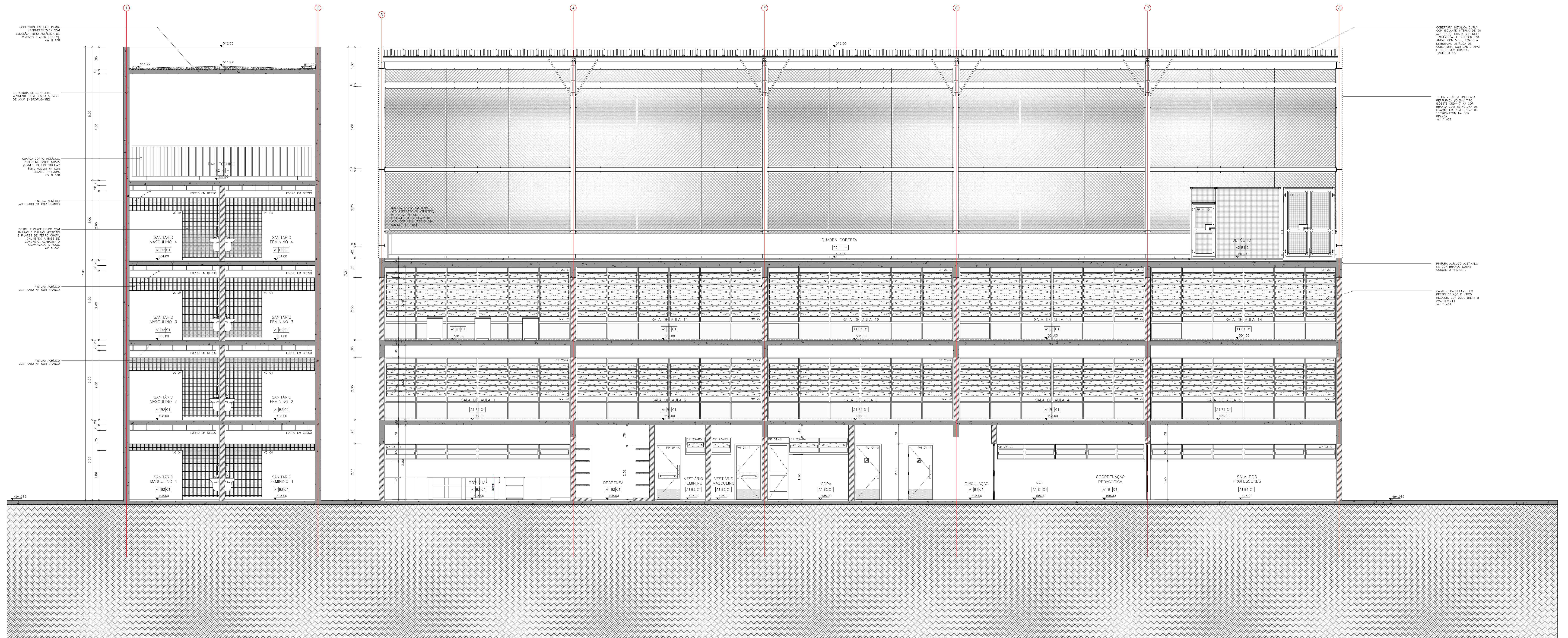
CORTE AA ESCALA 1:50
